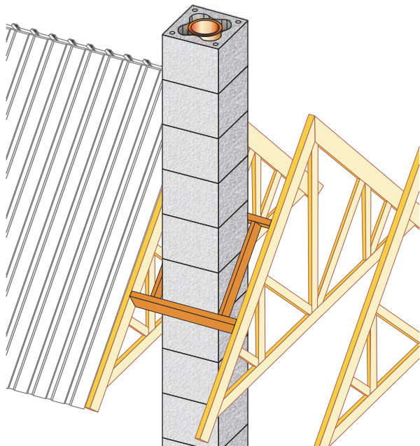
KUVA 1 Asenna piipun ympärille apukoolaukset 50 mm etäisyydelle piipun ulkopinnasta. Varmista etäisyys piipun valmistajalta.
