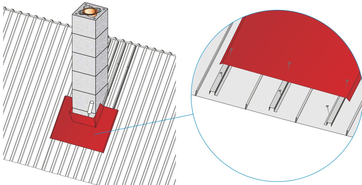
KUVA 5 Ennen asennuksen aloittamista poista pellityssarjan suojamuovi. Asenna alempi juuripelti kuvan mukaisesti käyttäen apuna rivipelti- ja konesaumakatoilla asennussarjan listoja (lisätarvike). Pursota tiivistemassaa piipun ja juuripellin ylösnostojen väliin.
