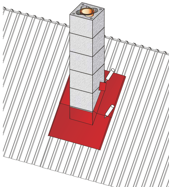
KUVA 7 Asenna ylempi juuripelti kuvan mukaisesti. Pursota tiivistemassaa piipun ja juuripellin ylösnoston sekä ylemmän ja alemman juuripellin liitoksiin.
