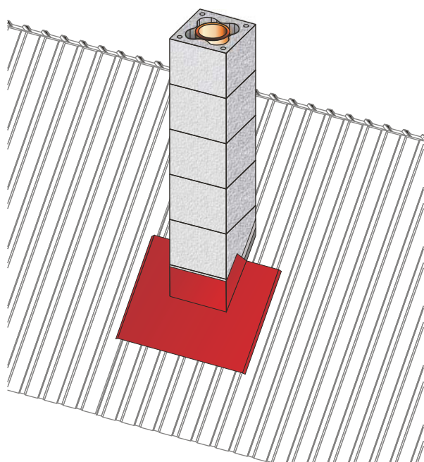
KUVA 6 Asenna alemman juuripellin säädettävä ylösnosto tiiviisti piippua vasten.
