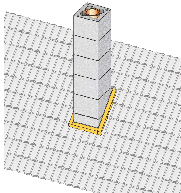
KUVA 4 Tiilikatossa kiinnitä apukoolaukseen kiinnitysrimat pellityssarjan kiinnittämiseksi vähintään 20 mm etäisyydelle piipun ulkopinnasta. Varmista etäisyys piipun valmistajalta. Kiinnitysrimat tulee asentaa tiilikaton kanssa samaan tasoon.
