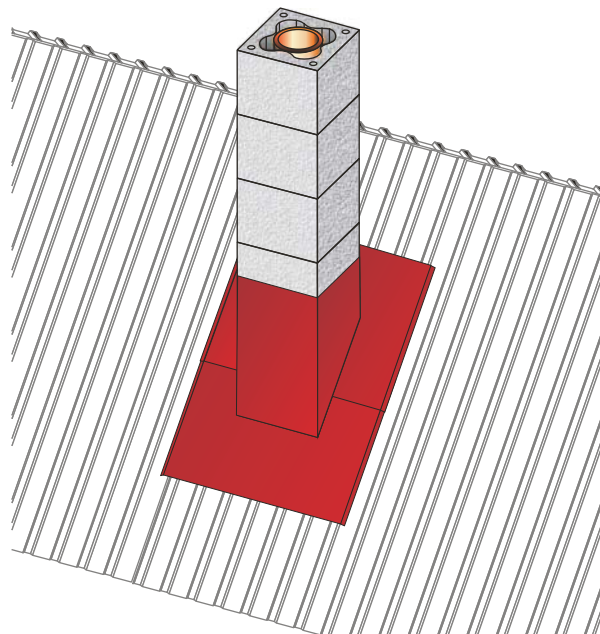
KUVA 10 Asenna lyhyempi vaippapelti paikoilleen siten, että juuripellin ylönostot jäävät vaippapellin sisäpuolelle.
