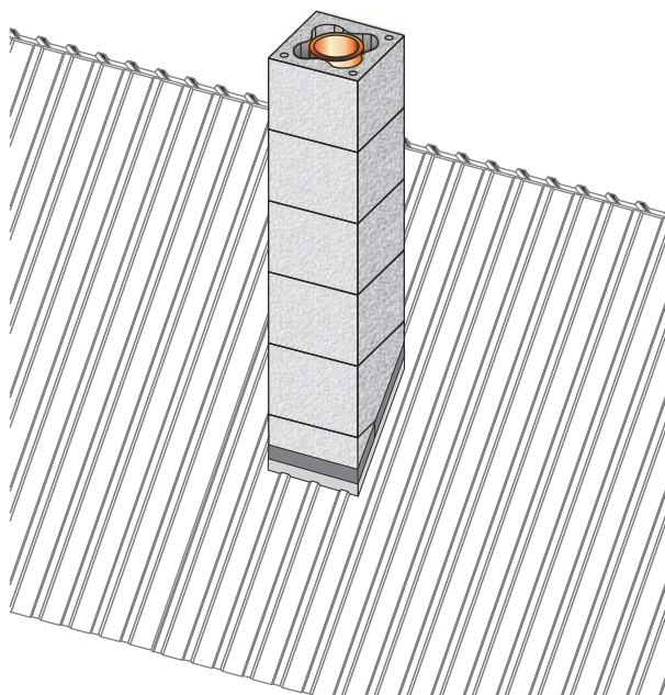
KUVA 3 Asenna vesikate.
