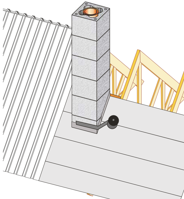
KUVA 2 Asenna aluskate piipun harjan puoleiseen reunaan saakka. Nosta aluskate piippua vasten n. 100 mm ja teippaa piipun juuri huolellisesti läpivientien tiivistyspakettilla (lisätarvike).
